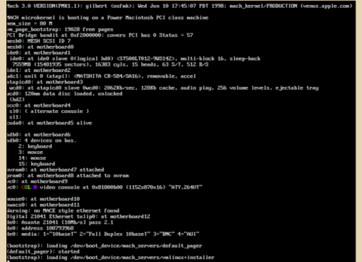
Рис 20. Ядро Mach 3.0 запускается с жёсткого диска и далее стартует уже сам Linux с компакт-диска
