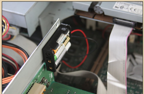
Рис 4. Неразборная батарейка PRAM-памяти Rayovac 840 давно села и заменена на «аналог» из 3 батареек AAA
