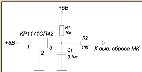
Рис. 3. Схема сброса с использованием КР1171СП42
